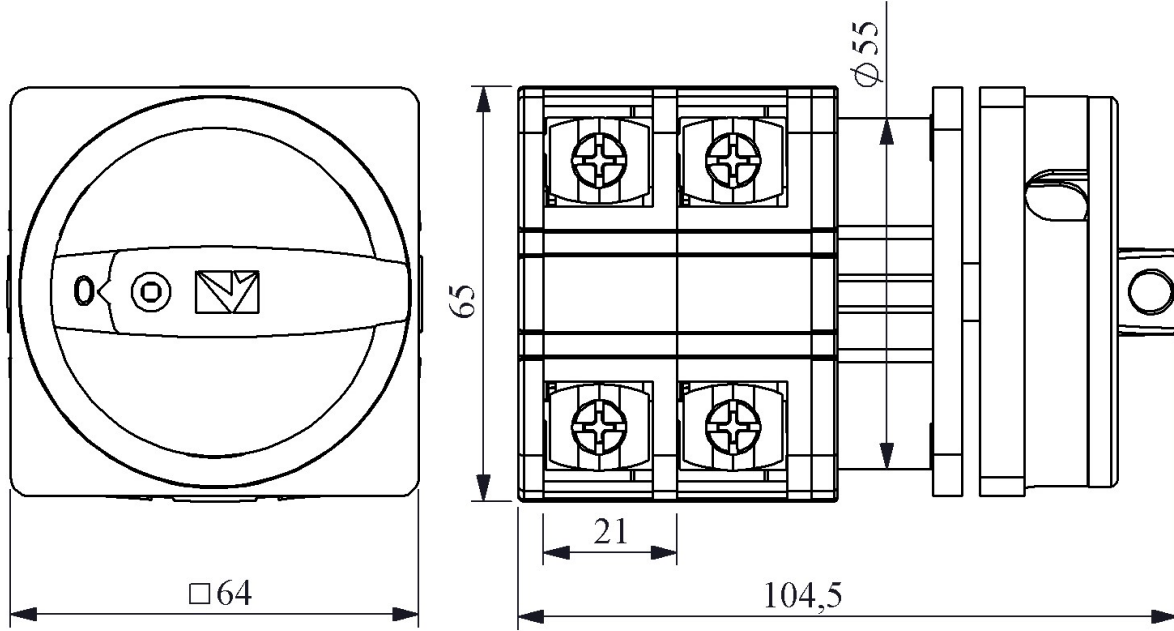
Devre Şeması
